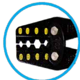
TP-38HB: 六角
